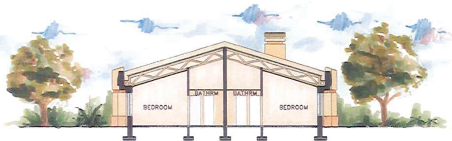
SECTION A-A Scale 1:100
